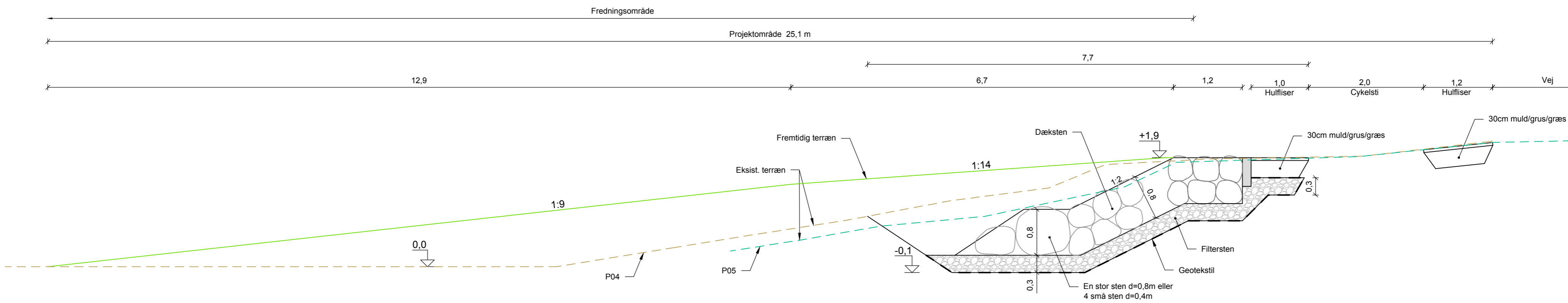
PRINCIPSNIT, 1:50
